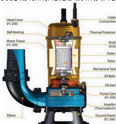
2.3.8 แสดงภาพตัวอย่างหลักการทำงานของปั๊มแช่ ไดโว่
