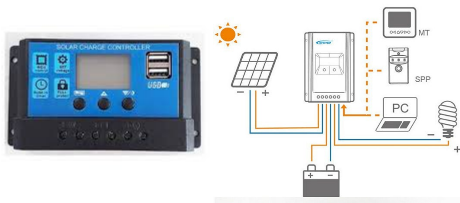
2.3.2.3 แสดงภาพตัวอย่าง ชาร์จเจอร์โซลาร์เซลล์ (Solar Charger)
