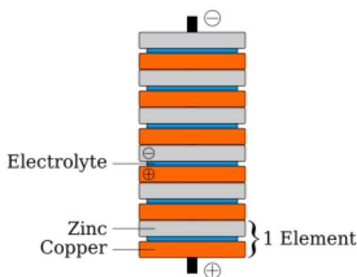
2.3.6.4 แสดงภาพส่วนประกอบของ Voltage pile
